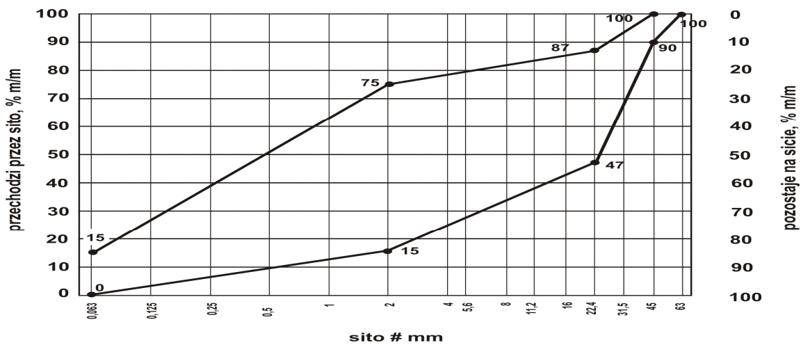
Rys. 18. Uziarnienie mieszanki niezwiązanej 0/31,5 dla nawierzchni
