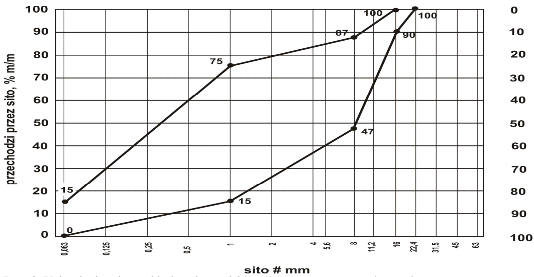
Rys. 3. Uziarnienie mieszanki niezwiązanej 0/16 dla warstwy mrozoochronnej
