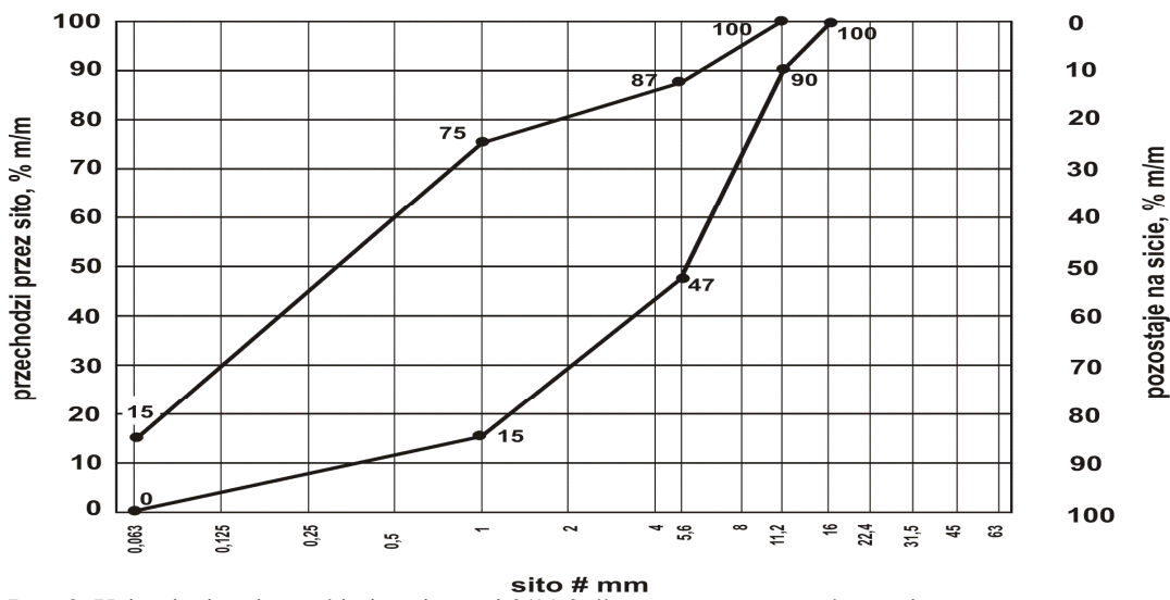
Rys. 2. Uziarnienie mieszanki niezwiązanej 0/11,2 dla warstwy mrozoochronnej
